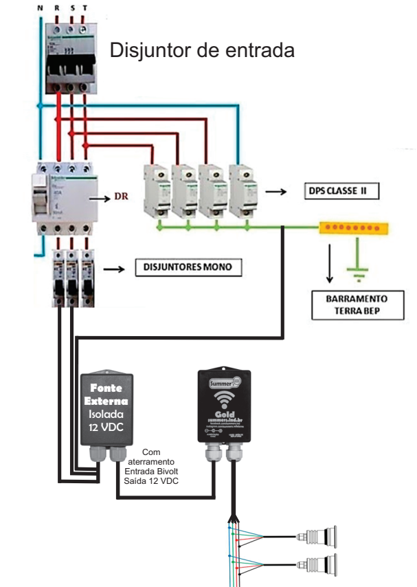
Esquema de ligação
